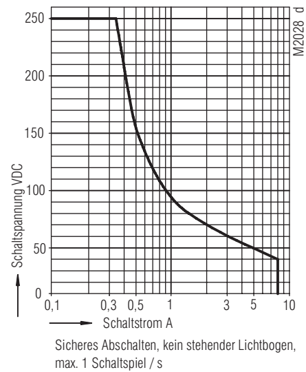
Lichtbogengrenzkurve (Sofortkontakte)
