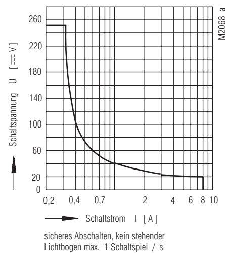
Lichtbogengrenzkurve (verzögerte Kontakte)
